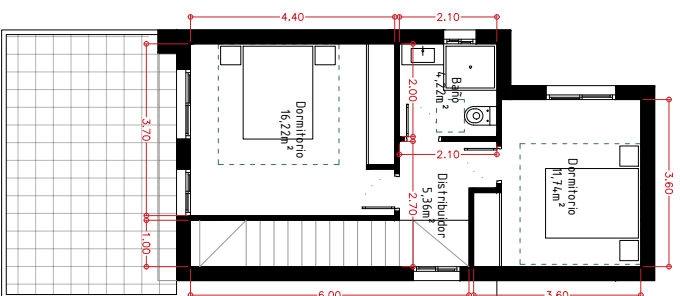
Planta Primera
