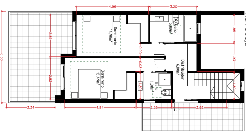
Planta Baja
