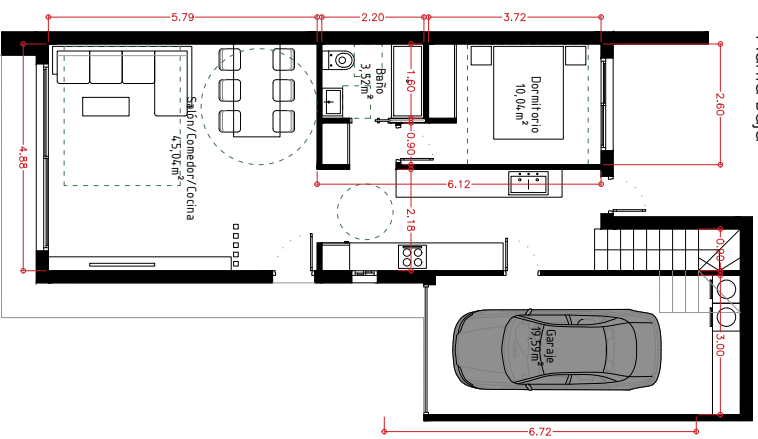
Planta Baja
