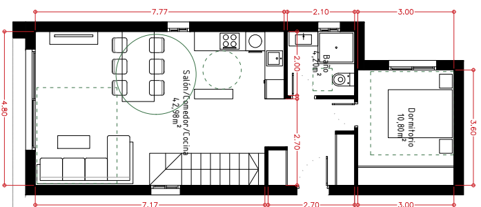
Vivienda Tipo C Planta Baja
