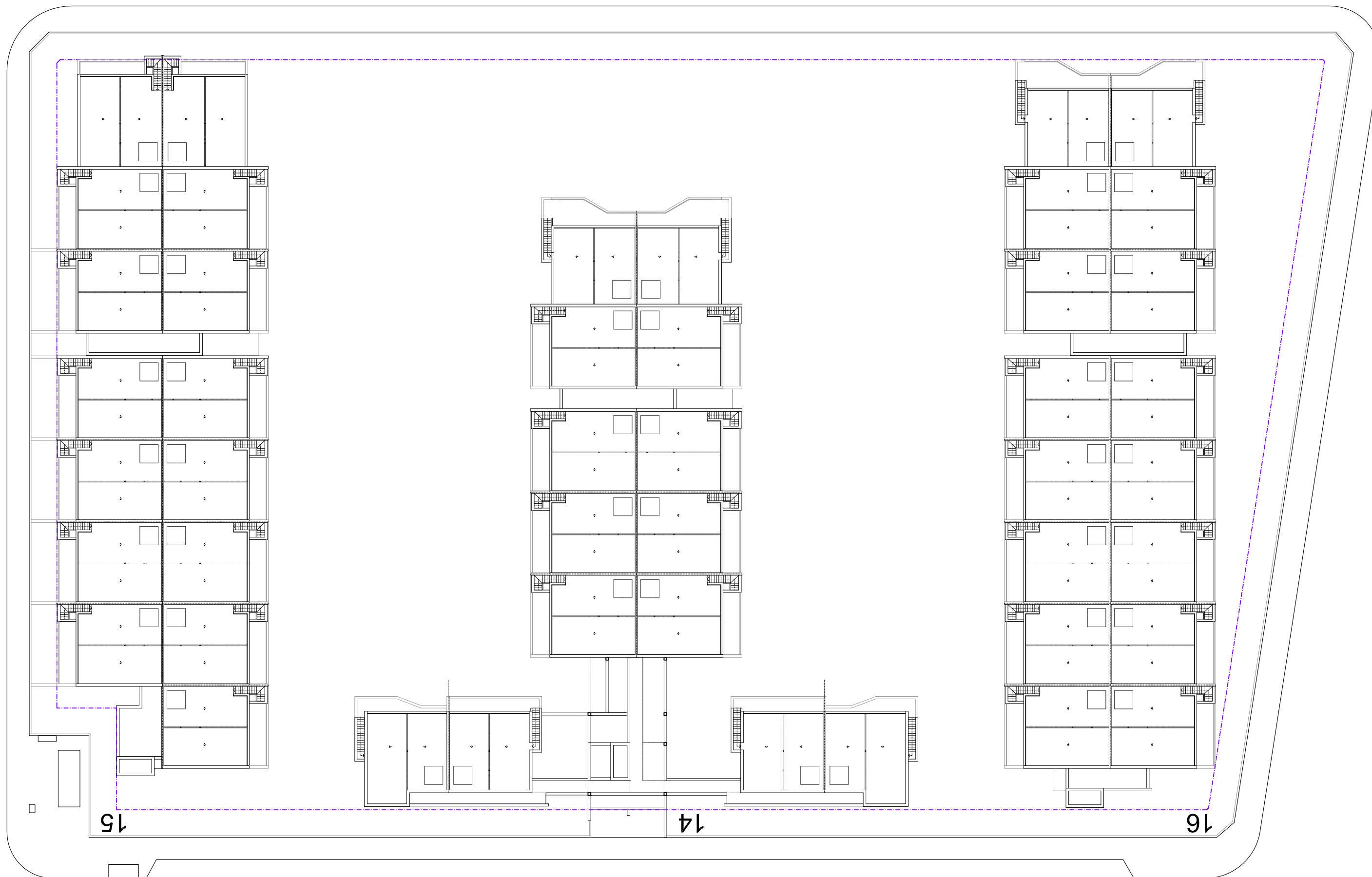
PLANTA CUBIERTA
